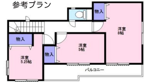
2F 42.23㎡ (12.77坪)
